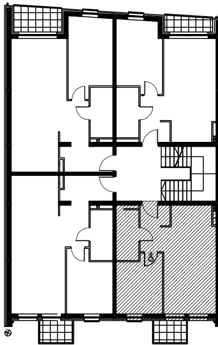
RZUT BUDYNKU PIĘTRO 2
