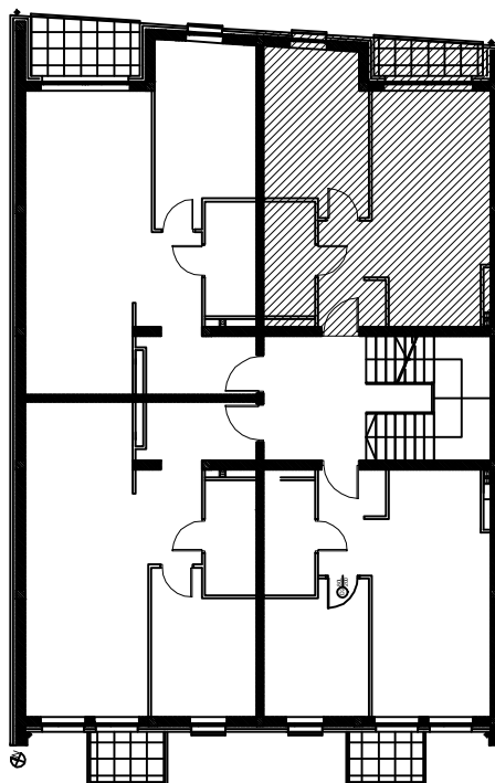
RZUT BUDYNKU PIĘTRO 3
