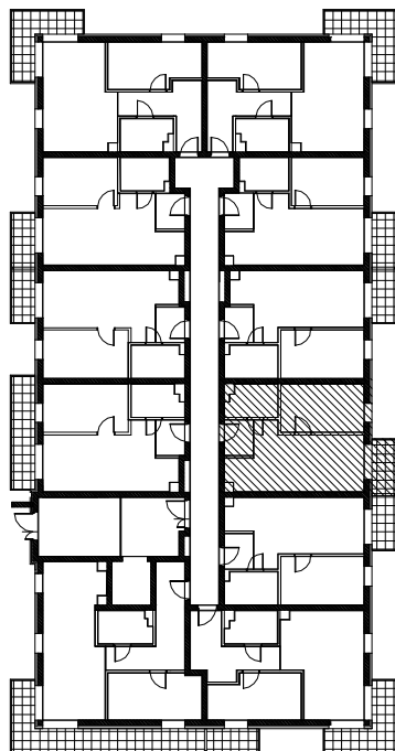
RZUT BUDYNKU PIĘTRO 1
